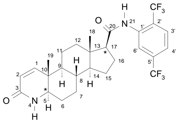
Dutasteride:
